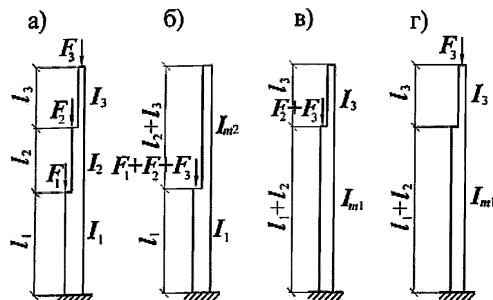
Рисунок II.1 – Схема двухступенчатой колонны (а) и условные схемы нагружений при приложении сил F_1 , F_2 и F_3 соответственно к нижнему (б), к среднему (в), к верхнему (г) участкам
